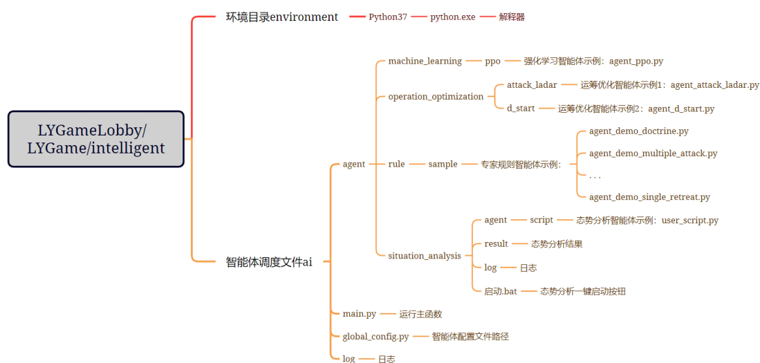
图 4 智能体使用文件结构
