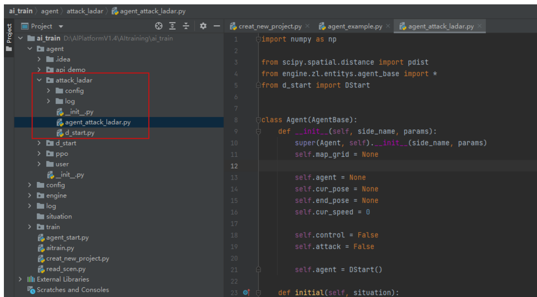
图 11 attack_ladar 工程
