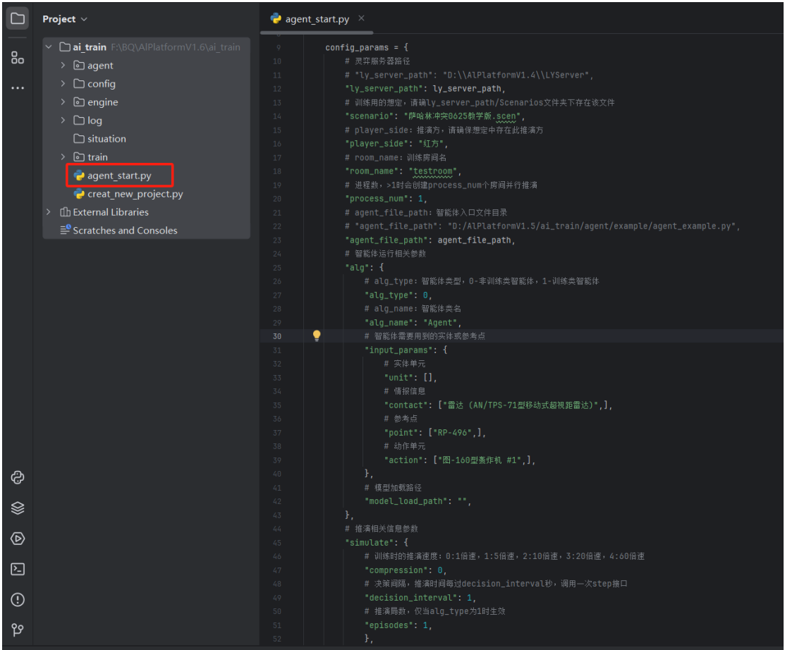
图 15 启动智能体配置项
