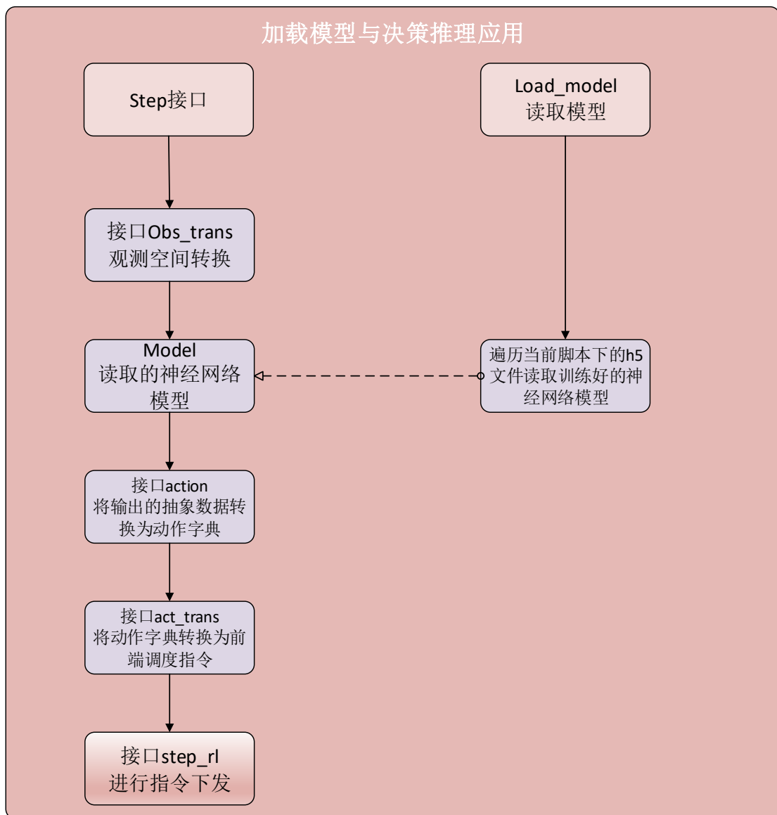
图 35 加载模型与决策推理应用
